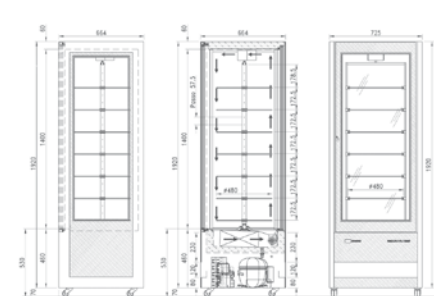
VISTA LATERALE
